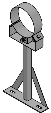
M 1:8 (Ø150)
