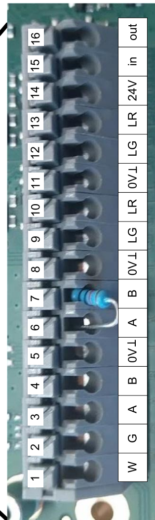
Klemmenbezeichnung
