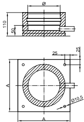
Grundplatte mit Kondensatablauf für Sockelmontage / DWETN66
