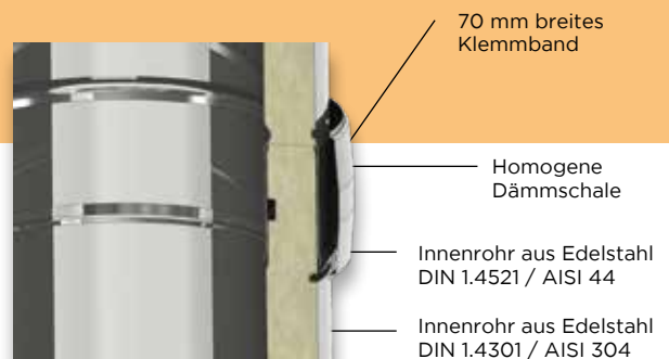
DW ECO 2.0 Standard Ausführung
