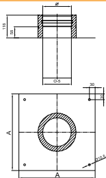
Grundplatte für Kaminerhöhung / DWETN08
