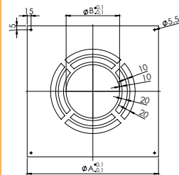
Deckenblende O° 1-teilig (hinterlüftet) / DWECO70HL
