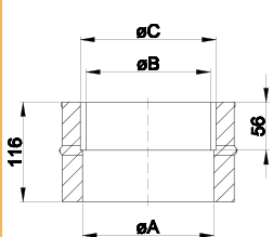
Übergang EW-DW mit integriertem Wandfutter, -gerade- / DWECO37GW
