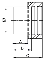
Übergang EW-DWECO / DWETN37
