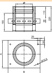
Grundplatte für Zwischenstütze / DWECO07
