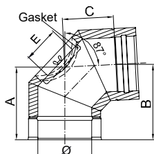
Winkel 87° / DWETN64
